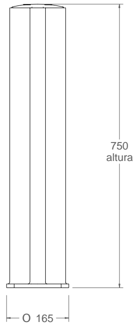
vista alzado 1:10
