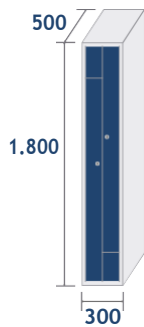
ECOL-30/1 PRO COD: 35301 24,4kg · 0,27m 3
