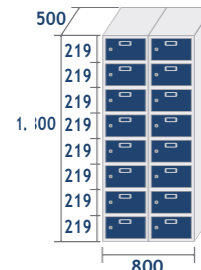
ECOZ-40/2 PRO COD: 47120 56,8kg · 0,72m 3
