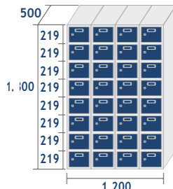
ECOZ-30/4 PRO COD: 47117 91,8kg · 1,08m 3
