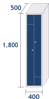
ECOL-40/1 PRO COD: 35401 28,1kg · 0,36m 3
